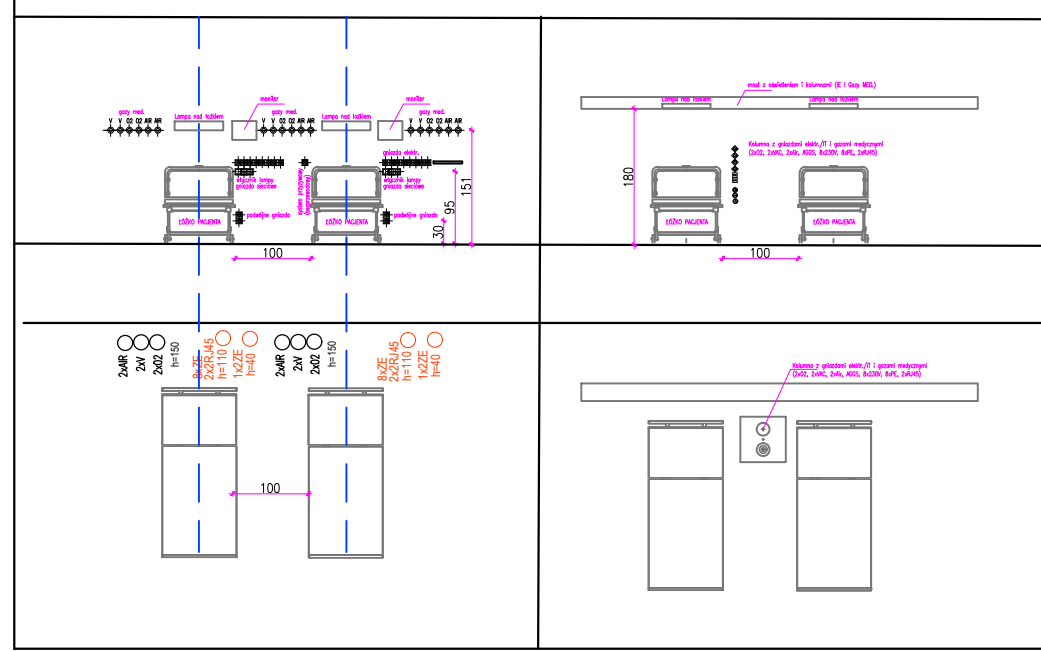
SCHEMAT ROZŁOKOWANIA GNAZD (ELEKTRYCZNYCH I GAZÓW MEDYCZNYCH) PRZY STANOWISKACH OBSERWACJI I NADZORU
